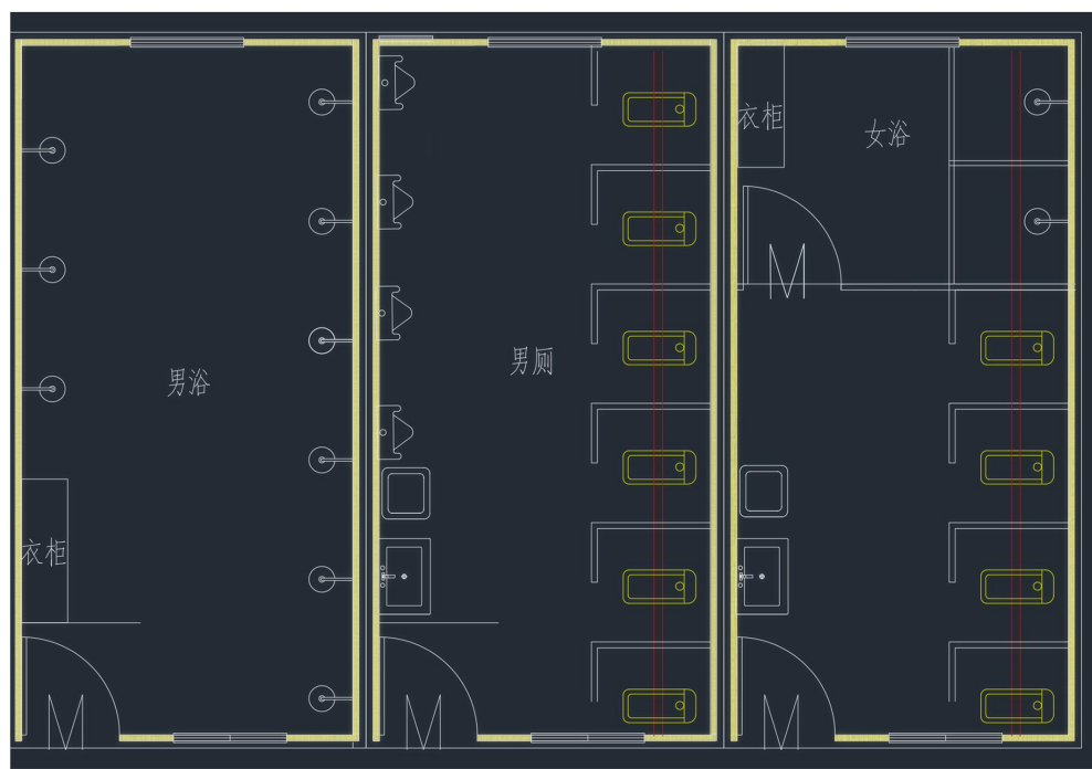
洗漱间详图
