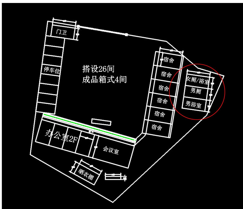
洗漱间详图
